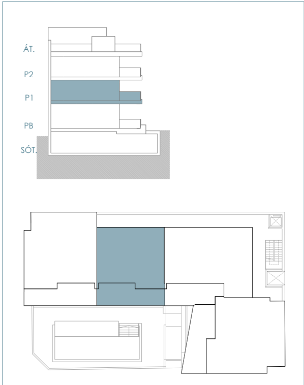
Planta Primera First Floor
